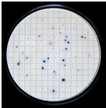
Filtrierte Mischkultur von Escherichia coli , Enterobacter aerogenes und Pseudomonas aeruginosa nach 21 Stunden bei 37 °C.
